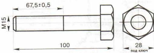
Рис. 2.3. Чертеж болта
